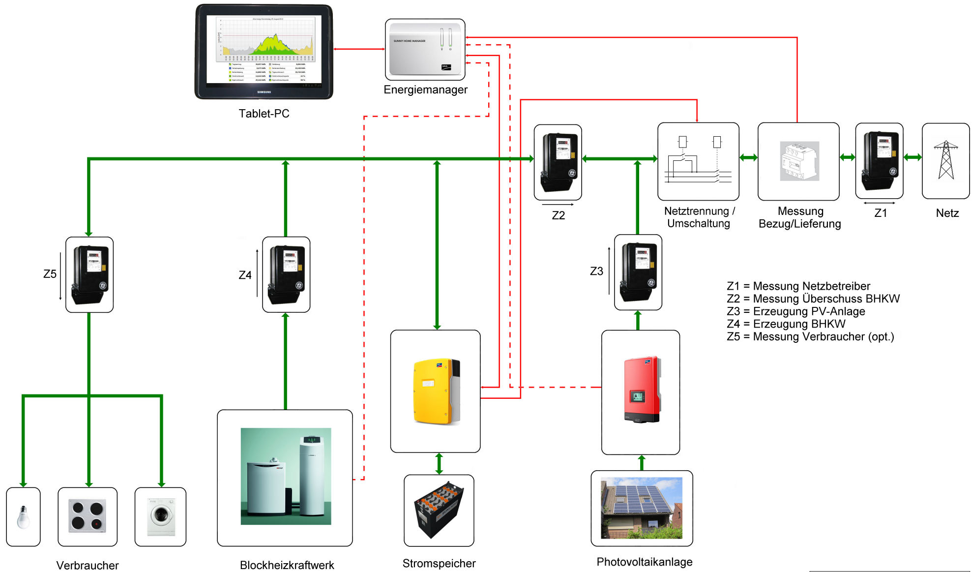
Prinzipschaltbild Stromspeicher für Eigenverbrauchsoptimierung mit Notstromfunktion
